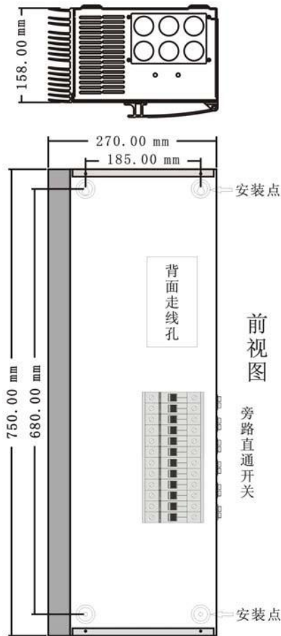
安装尺寸图
